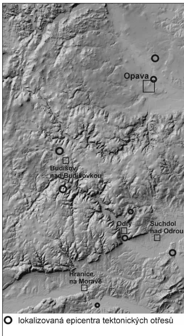
Epicentra lokalizovaných mikrozemětřesení z širší oblasti Poodří zaznamenaná od r. 1997.
